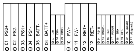
CONNETTORE su SCHEDA TD571
